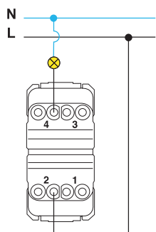
Одноклавишный выключатель
