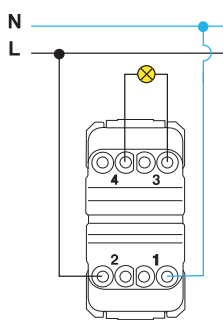
Двухполюсный выключатель
