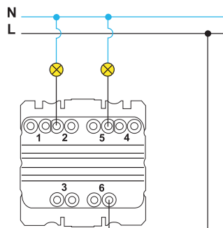
Двухклавишный выключатель
